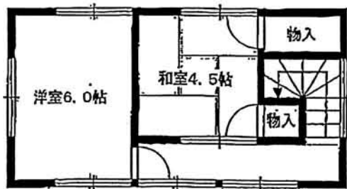
2階平面図
